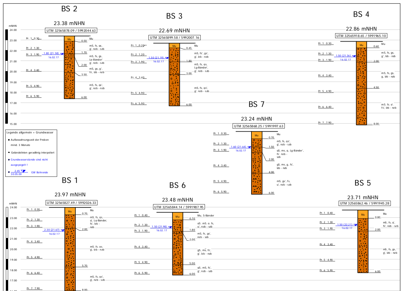
Abb. 4: Bodenprofile (Ausschnittkopie Anl. 1.1), o. M.
